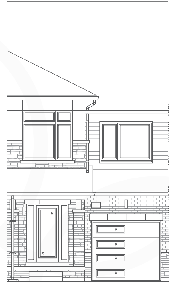
ELEVATION 1B
